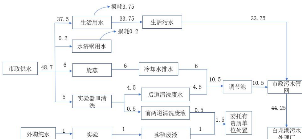
图 2-1 本项目水平衡示意图（单位：t/a）
