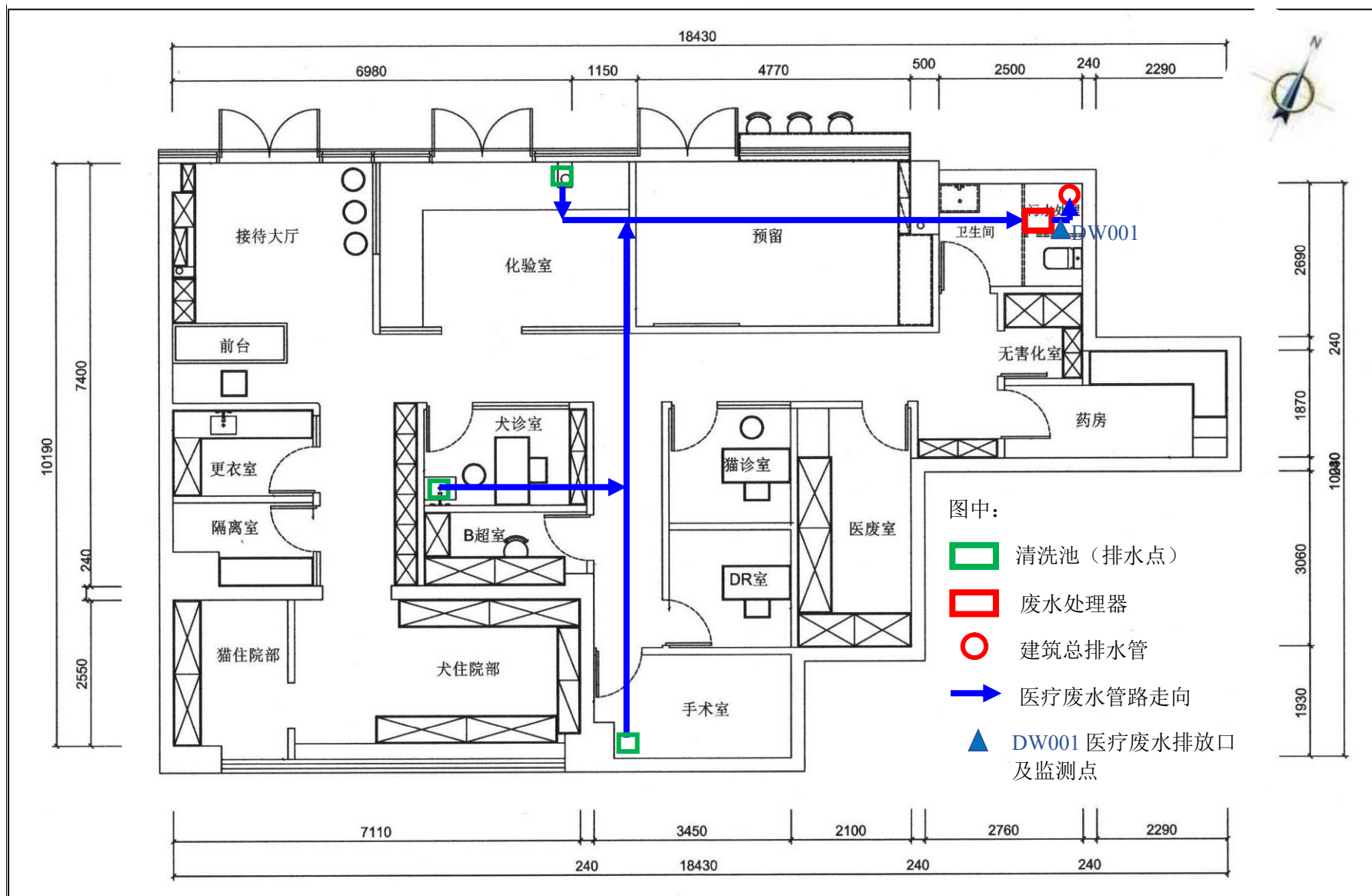
附图2 项目排水系统图
