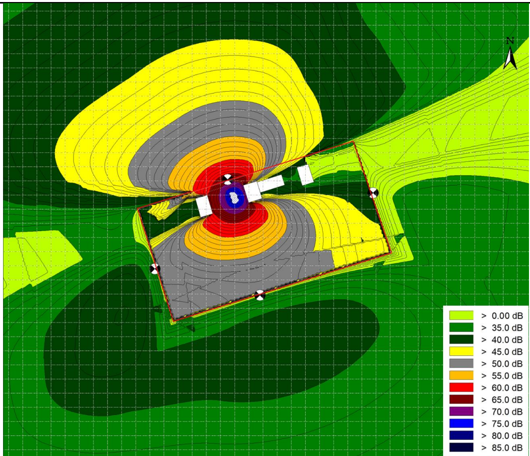
图 4.4-3 变压器噪声影响预测结果(预测高度 1.5m)(图示网格线为 10m*10m)
