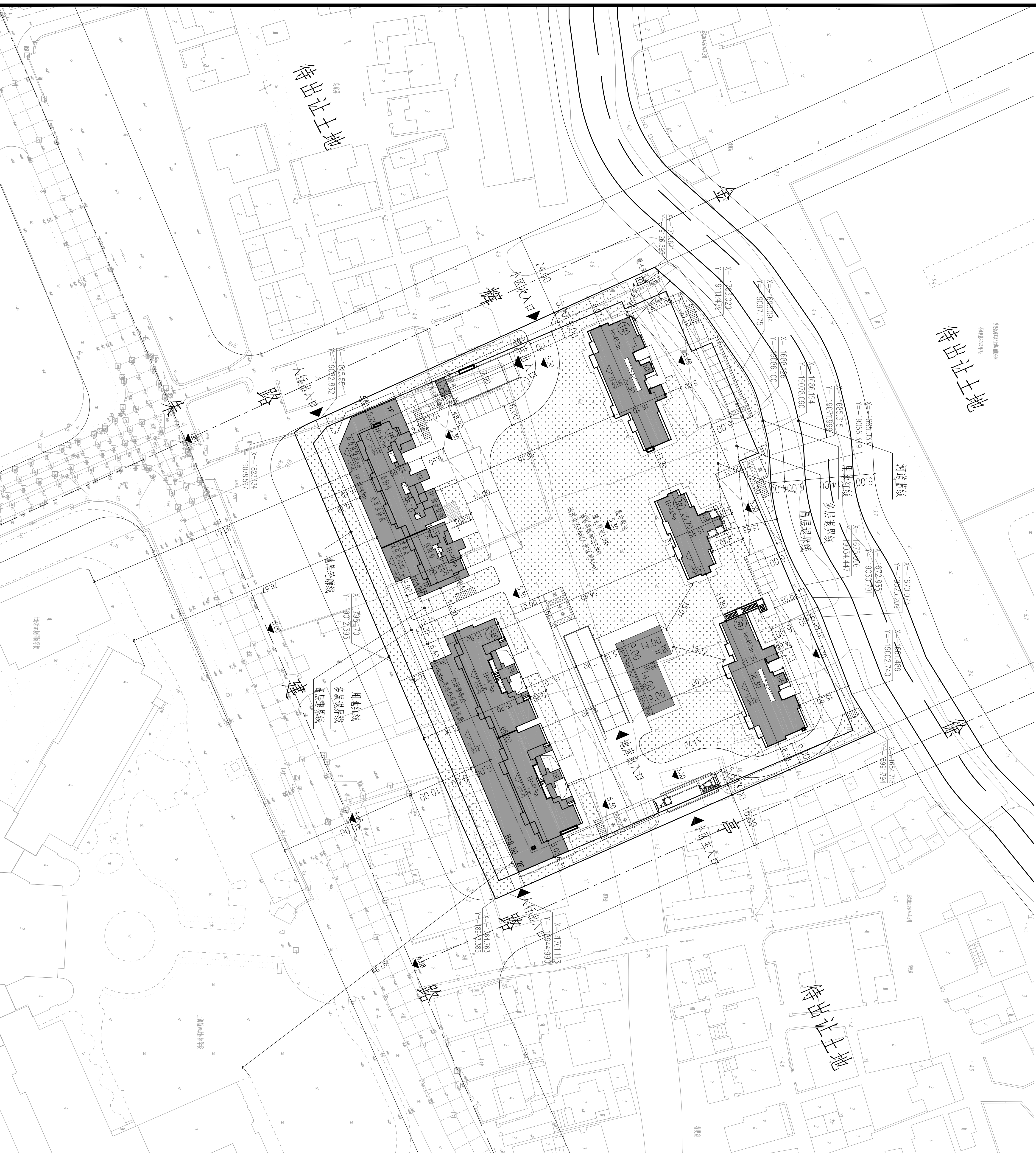
总平面图 1:500
