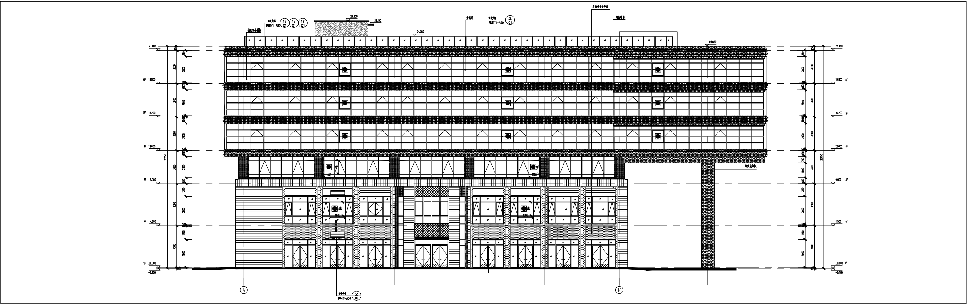
2#东立面
