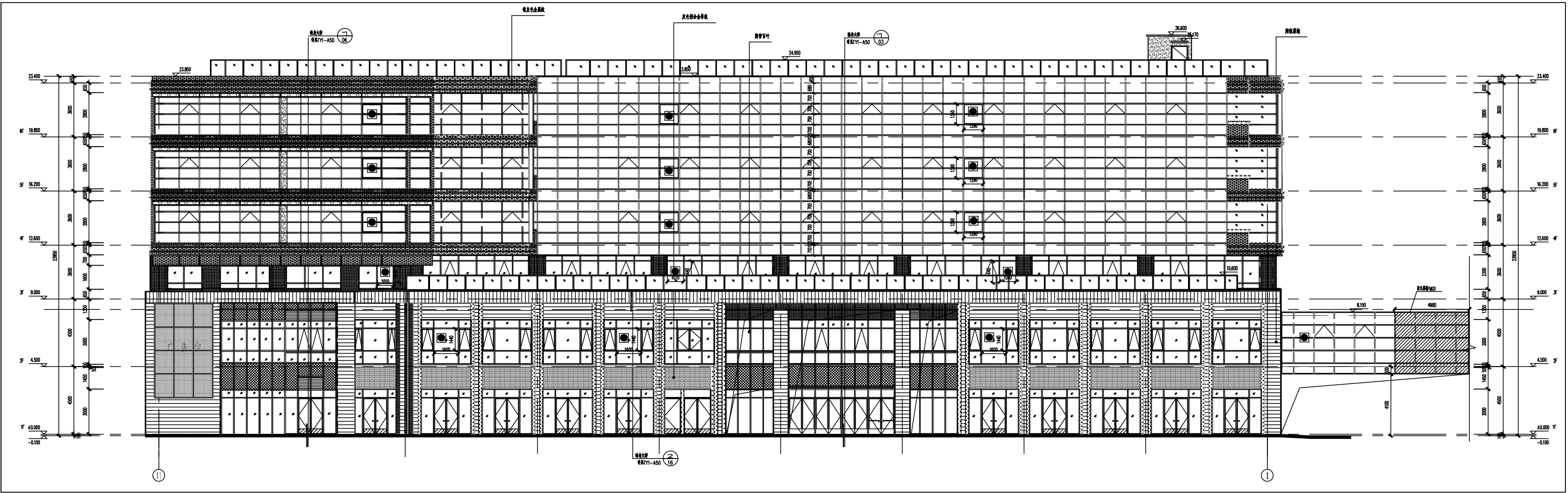
2#北立面
