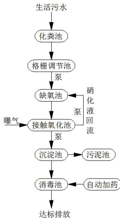
图5-1：污水处理工艺流程图
