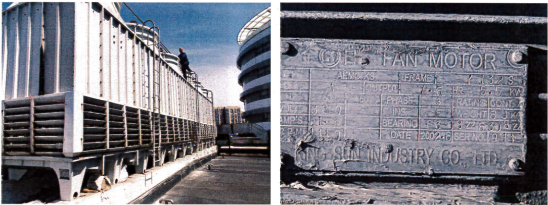
图 2.2-3 冷却塔组现场照片
