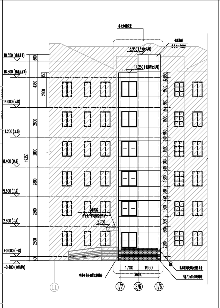
北立面图 1:100
