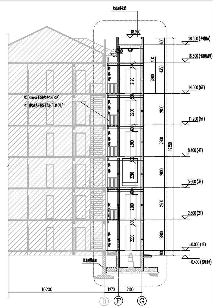
1-1剖面图 1:100
