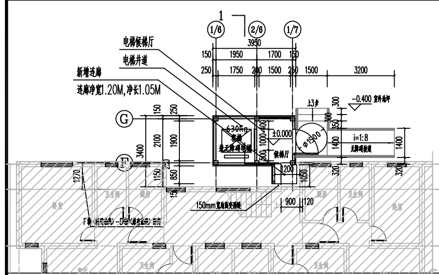
一层平面图 1:100
