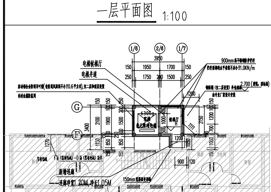
标准层平面图 1:100
