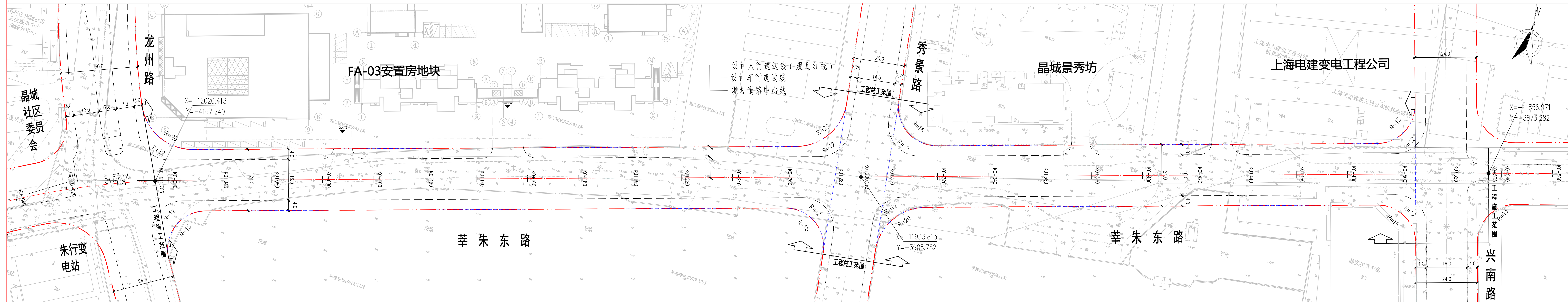
莘朱东路（龙州路-兴南路）道路平面图
