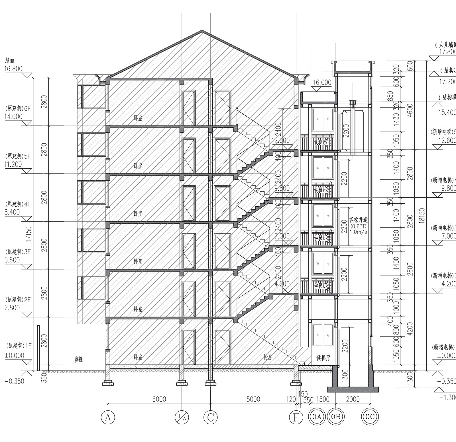
C-C剖面图
