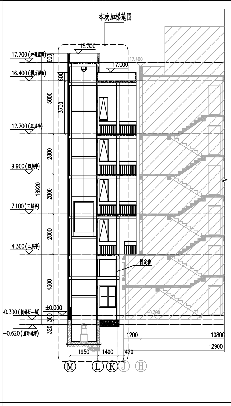
剖面图
