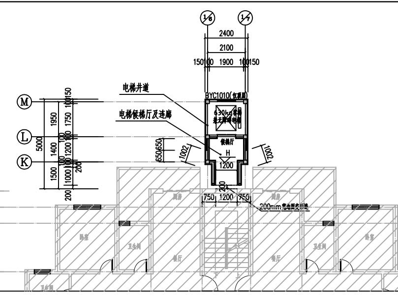
标准层平面图
