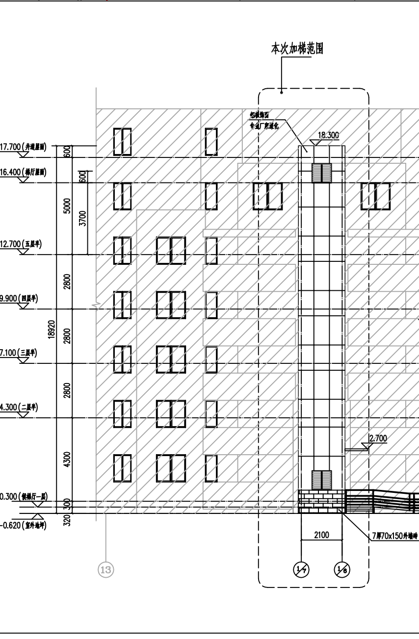
电梯北立面图
