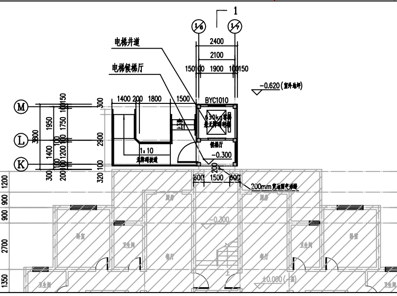
一层平面图
