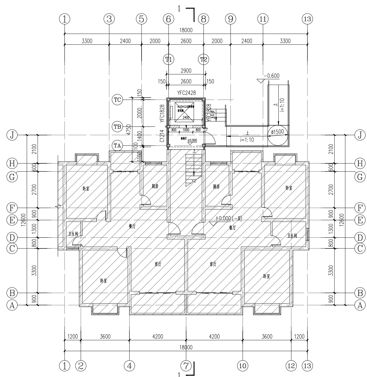
加梯后一层平面图
