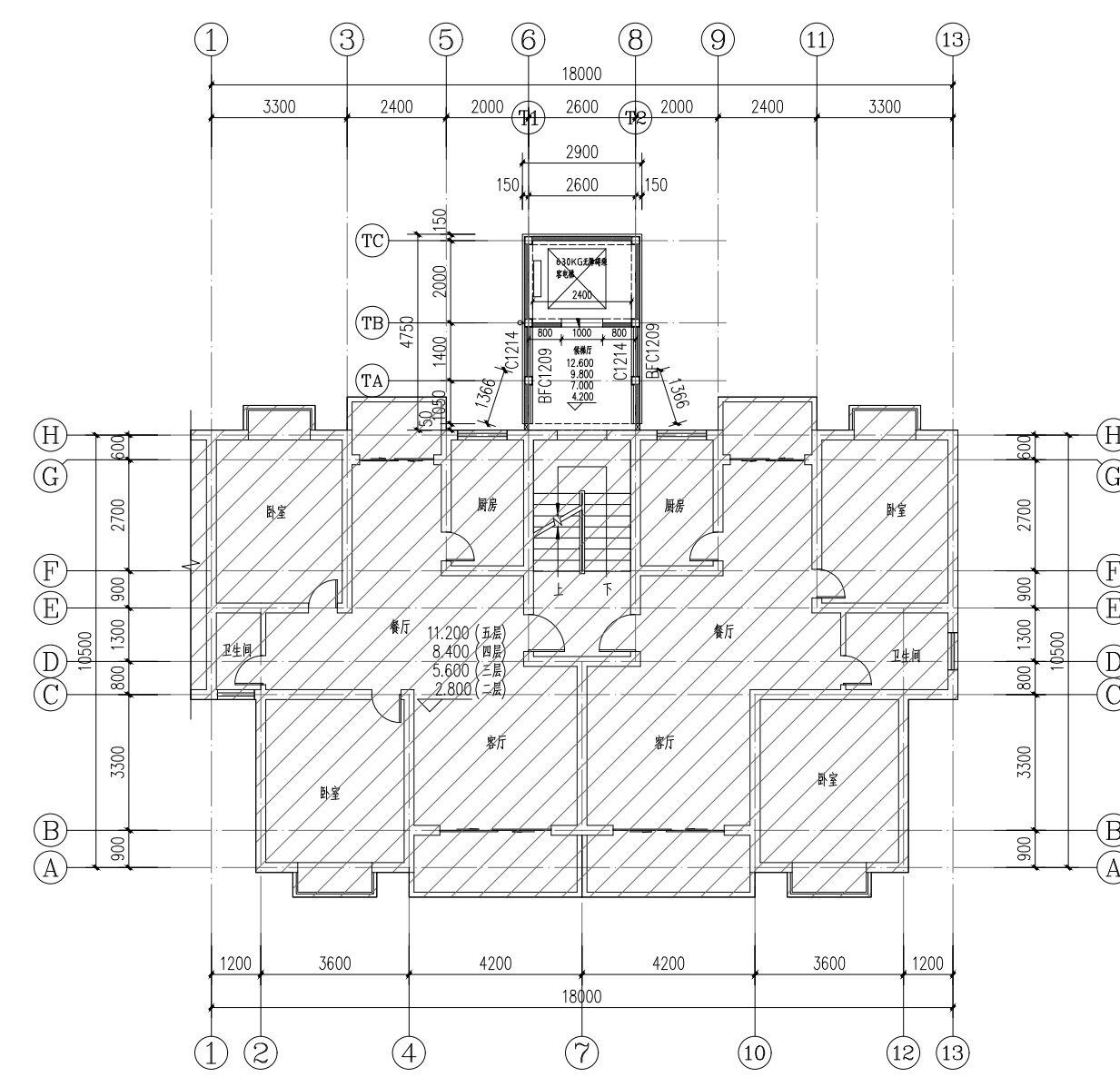
电梯标准层平面图
