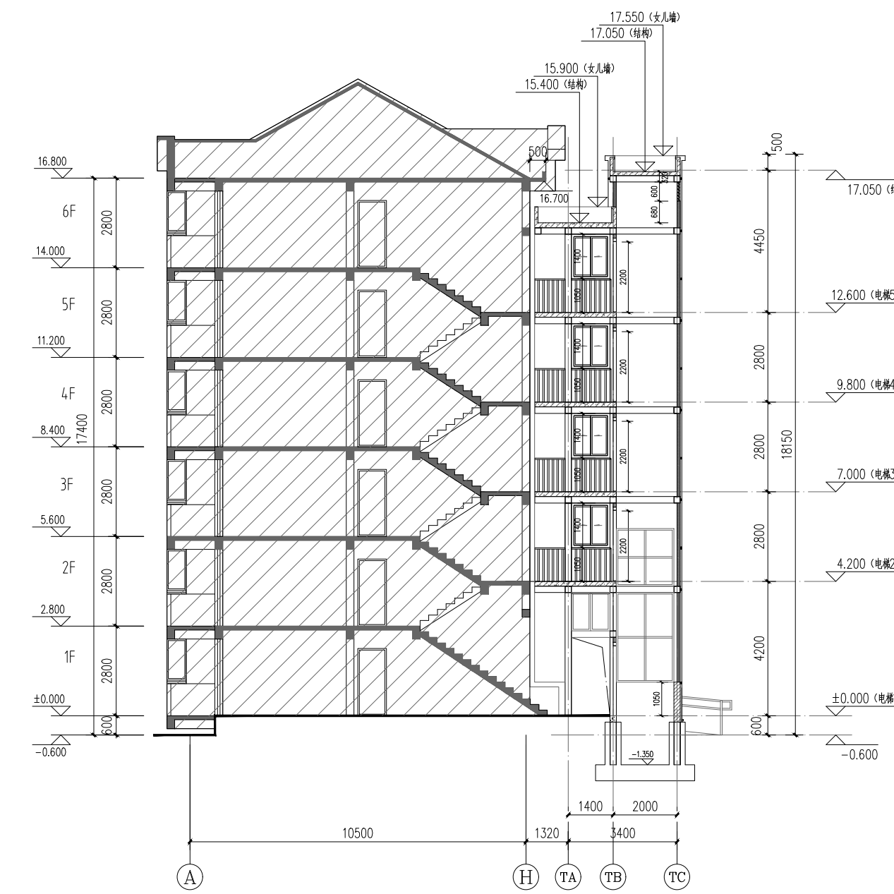
1-1剖面图
