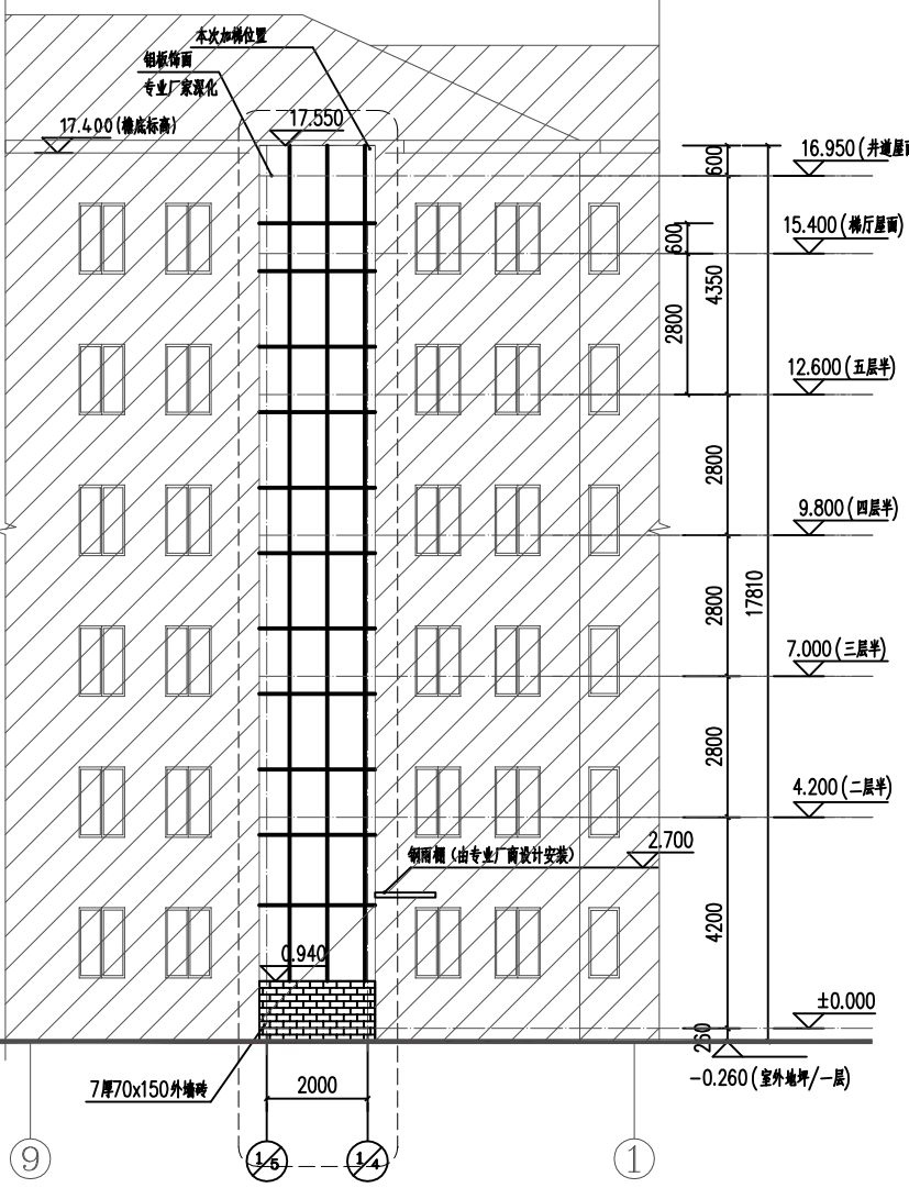
北立面图 1:100
