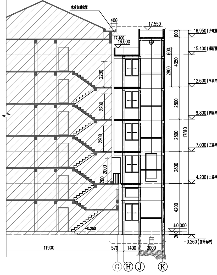
1-1剖面图 1:100
