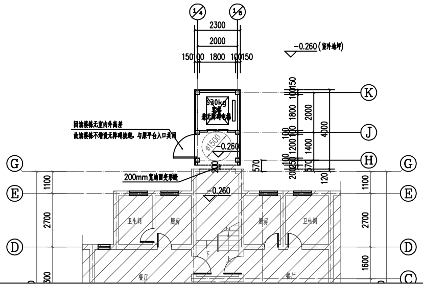
一层平面图 1:100
