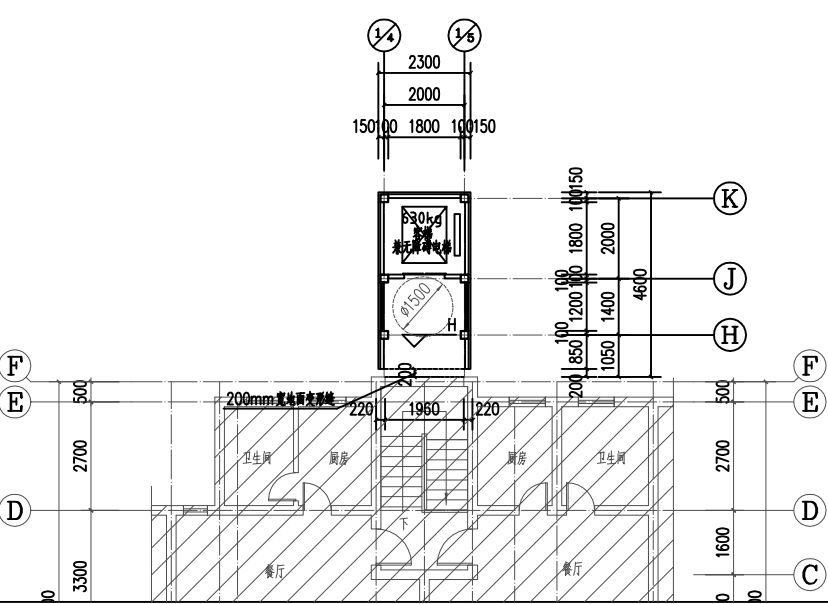
标准层平面图 1:100
