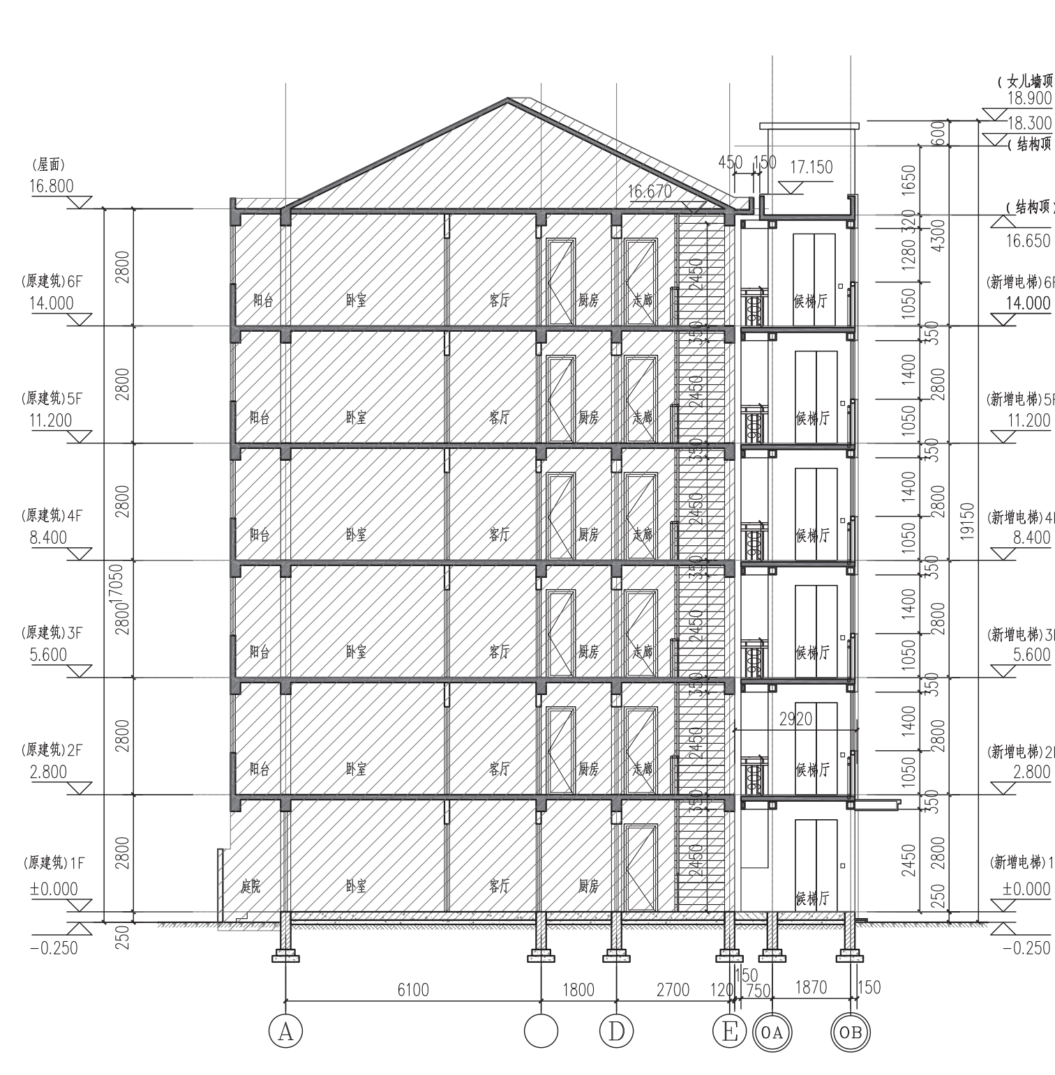
1-1剖面图
