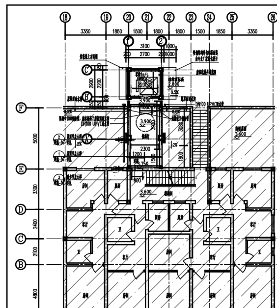
二层平面图
