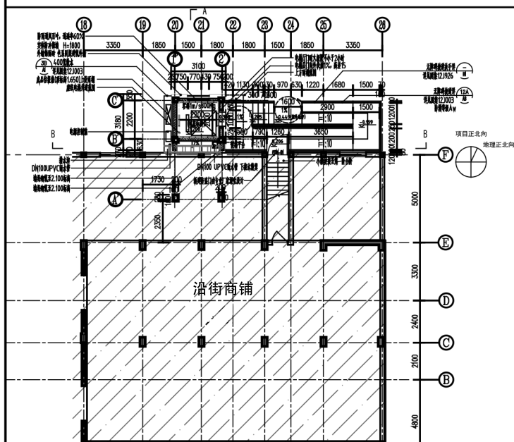
一层平面图
