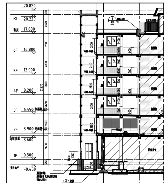
电梯剖面图
