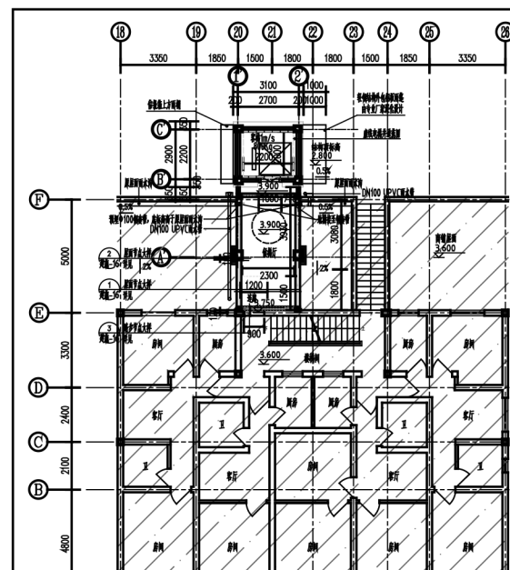
标准层平面图
