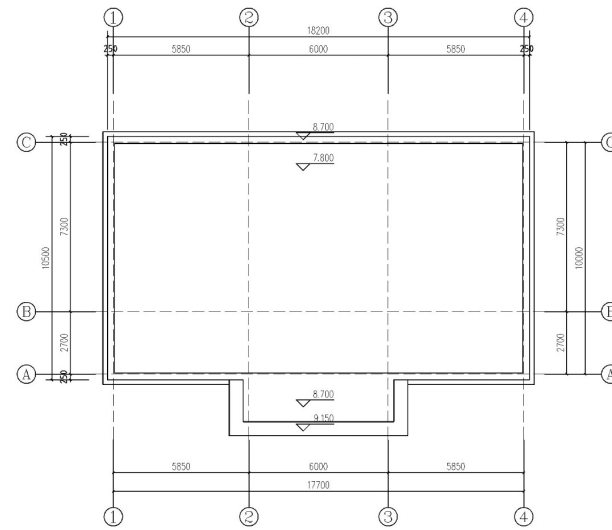
屋顶平面图 1:100
