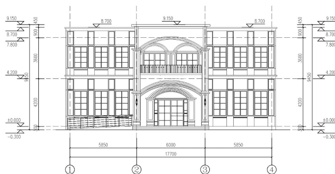
南立面图 1:100
