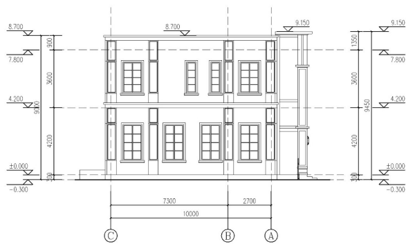
西立面图 1:100
