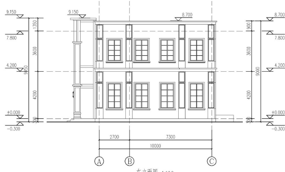
东立面图 1:100
