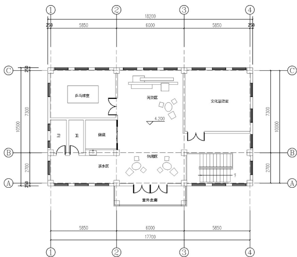
二层平面图 1:100
