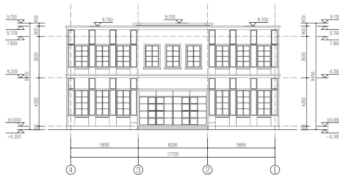
北立面图 1:100
