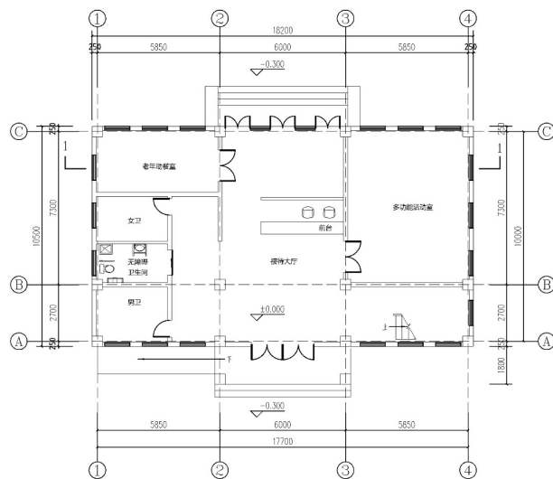
一层平面图 1:100
