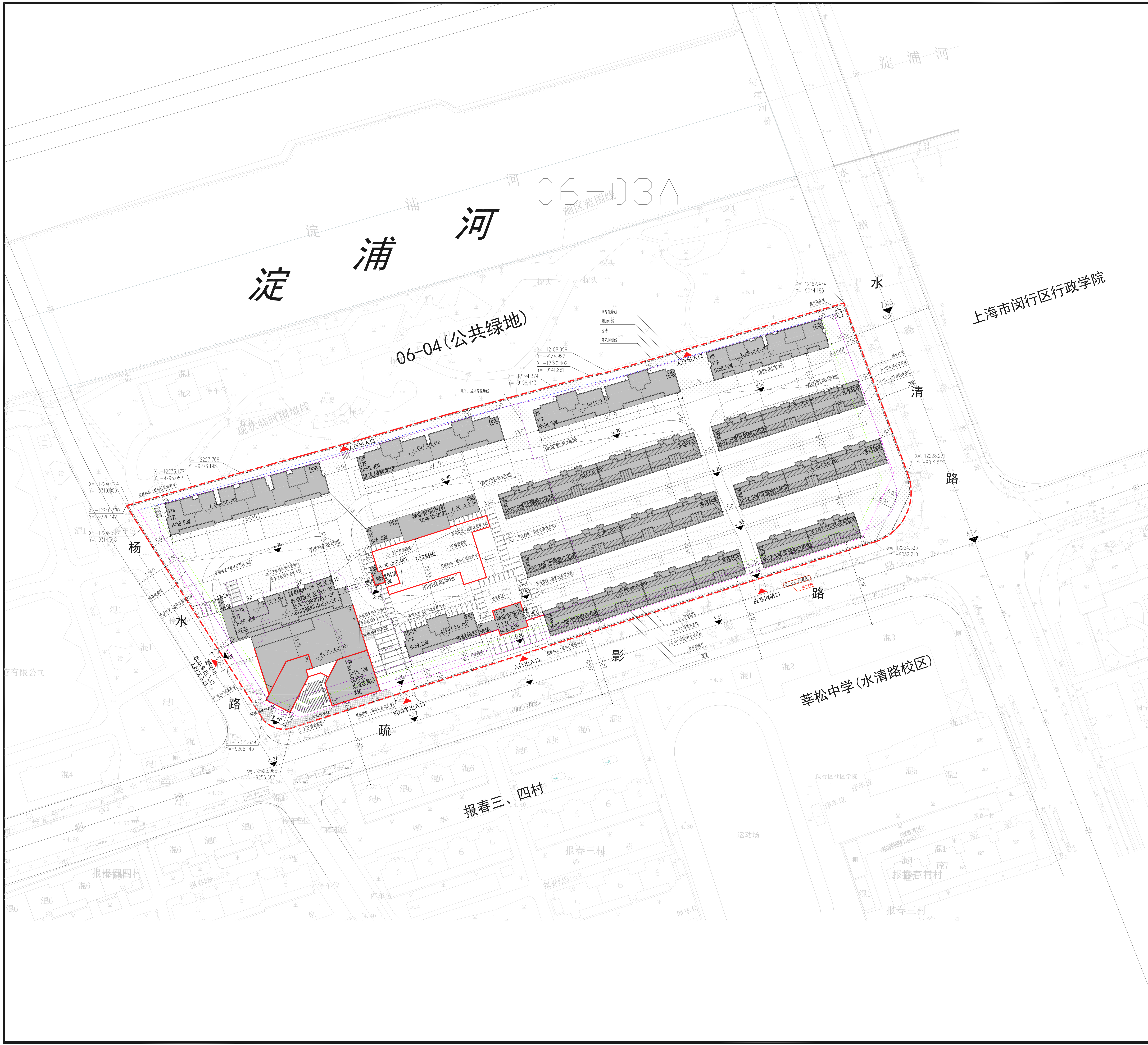
闵行区莘庄社区02单元06-05地块 住宅项目方案公示图
