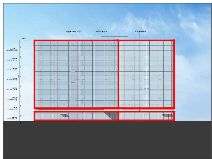
东立面图
