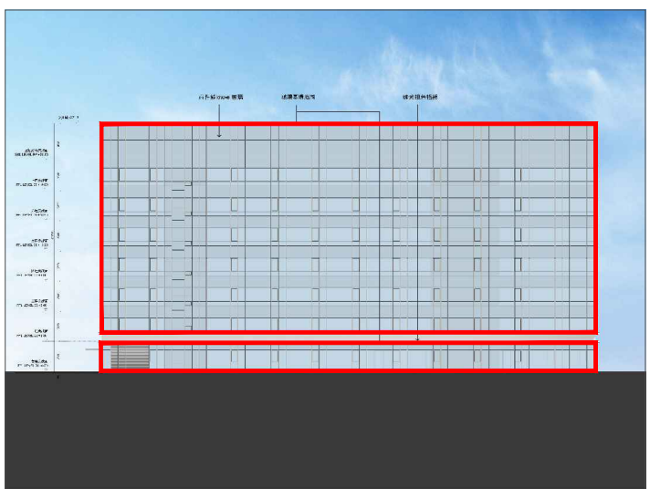
西立面图
