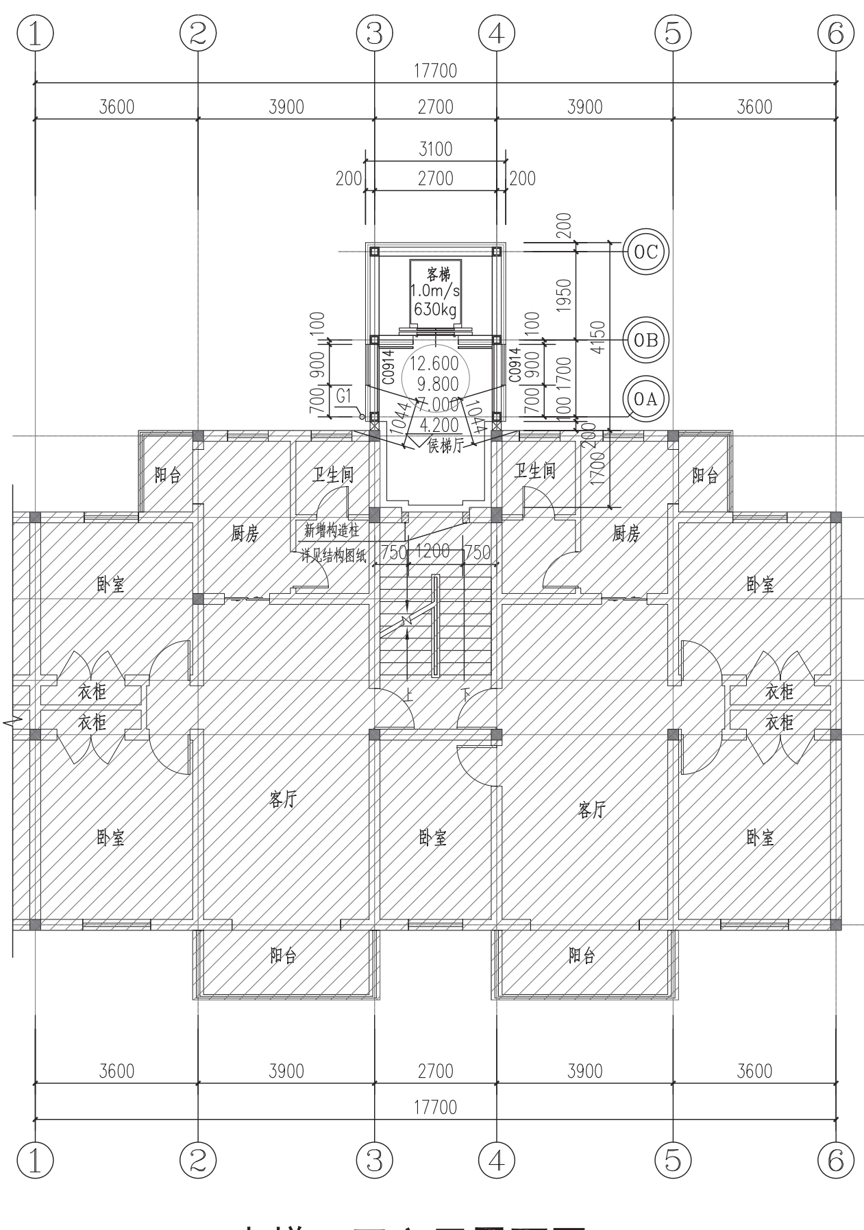
电梯二至六层平面图
