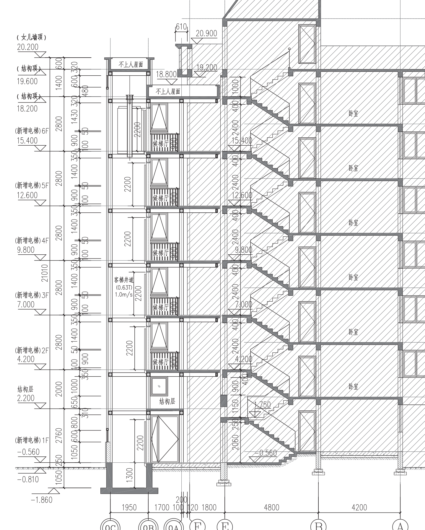
1-1剖面图
