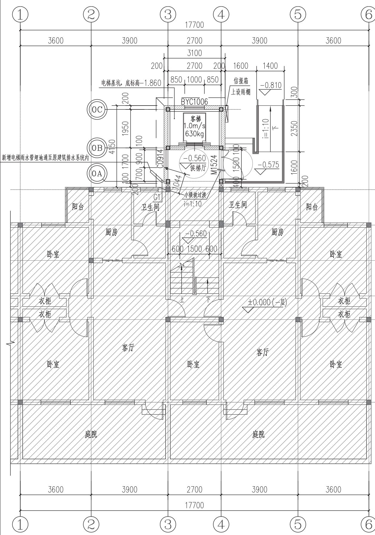
电梯一层平面图
