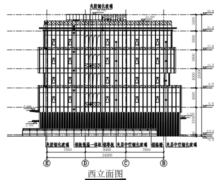
西立面图
