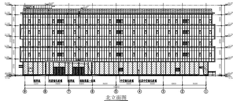
北立面图
