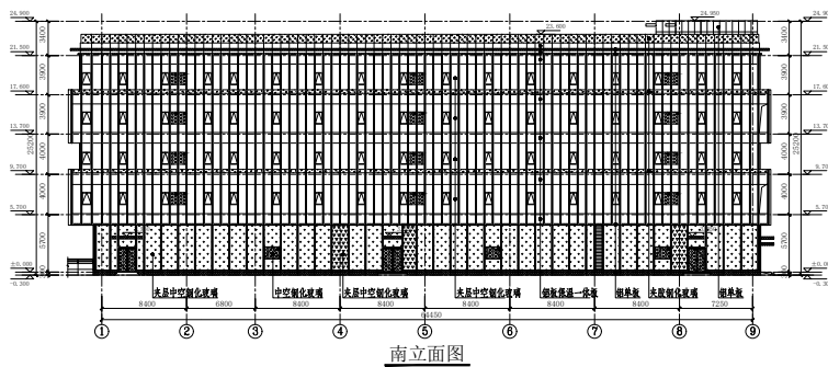
南立面图
