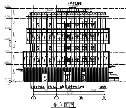
东立面图
